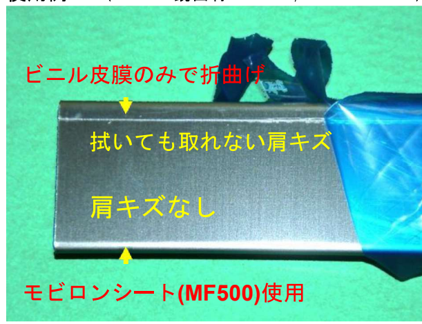
使用例 1 (SUS430 鏡面材 1.2t P/D=88° V=10 mm)
